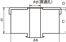
吊防振ゴム(W5/8・3/4)
