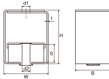
吊防振ゴムセット シングル(W5/8・3/4)
