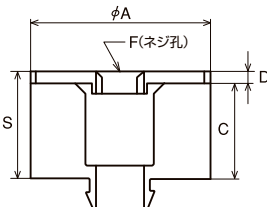
吊防振ゴム(W3/8・1/2)
