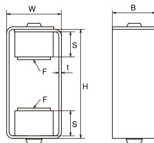
吊防振ゴムセット ダブル(W3/8・1/2)
