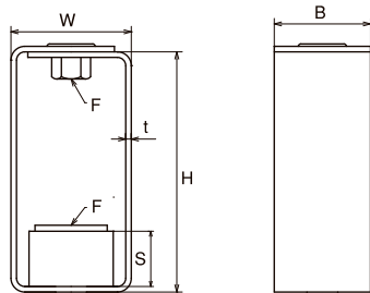
吊防振ゴムセット シングル(W3/8・1/2)
