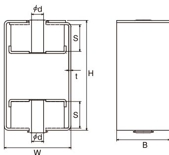
吊防振ゴムセット ダブル(W5/8・3/4)
