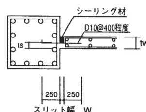
b) 部分スリット型の例
