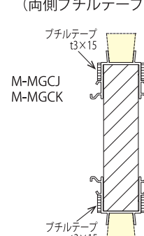
⑮鉛直X2 B3W (両側ブチルテープ付)
