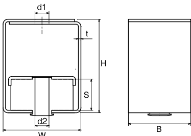
吊防振ゴムセット シングル (W5/8・3/4)
