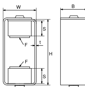
吊防振ゴムセット ステンレス ダブル(W3/8・1/2)
