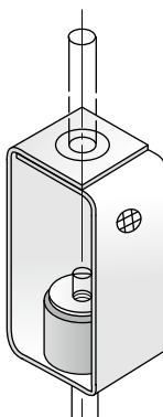
シングル仕様 (S) 施工状態 (W3/8・W1/2)
