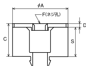
吊防振ゴム (W3/8・W1/2)
