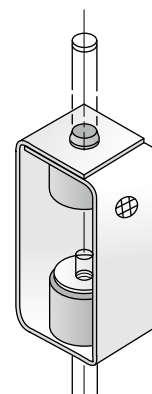
ダブル仕様 (D) 施工状態 (W3/8・W1/2)
