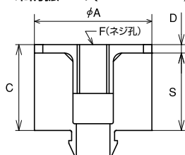
吊防振ゴム (W3/8・1/2)
