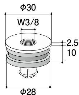
吊防振ゴム ミニ
