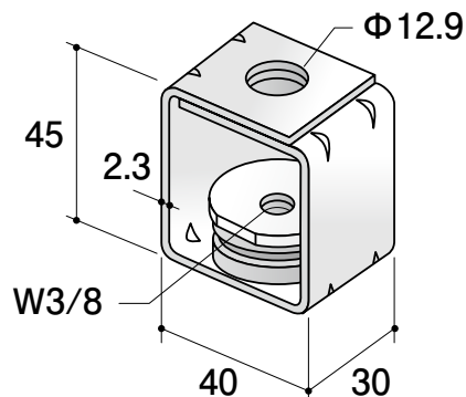
吊防振ゴムセット ミニ
