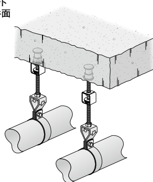
吊防振ゴムセット ミニ ナット付
