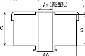
吊防振ゴム (W5/8・W3/4)
