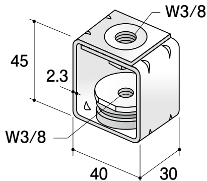
吊防振ゴムセット ミニ ナット付
