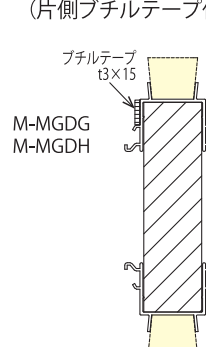
⑲鉛直X3 B3S (片側ブチルテープ付)
