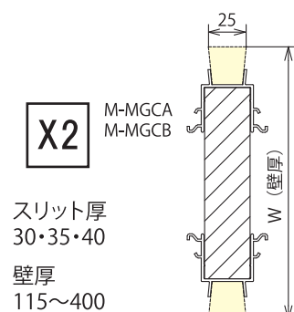
⑪鉛直X2タイプ
