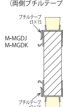
⑳鉛直X3 B3W (両側ブチルテープ付)
