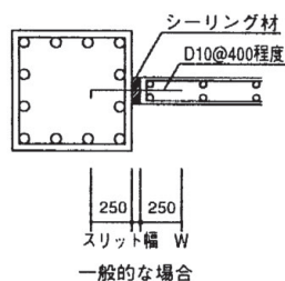
a) 完全スリット型の例
