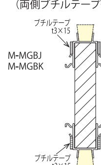
⑩鉛直X1 B3W (両側ブチルテープ付)
