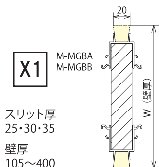
⑥鉛直X1タイプ
