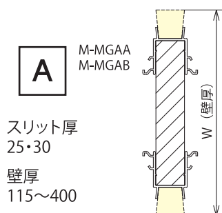
①鉛直Aタイプ
