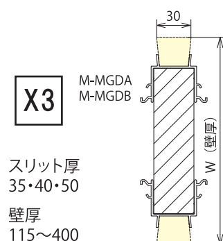
⑯鉛直X3タイプ
