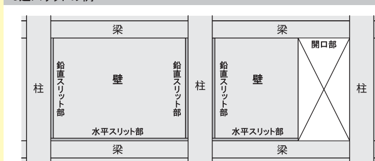
3辺スリットの例
