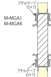
⑤鉛直A B3W (両側ブチルテープ付)
