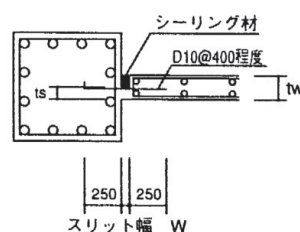
b) 部分スリット型の例
