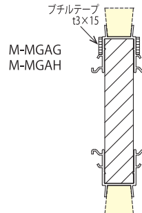
④鉛直A B3S (片側ブチルテープ付)
